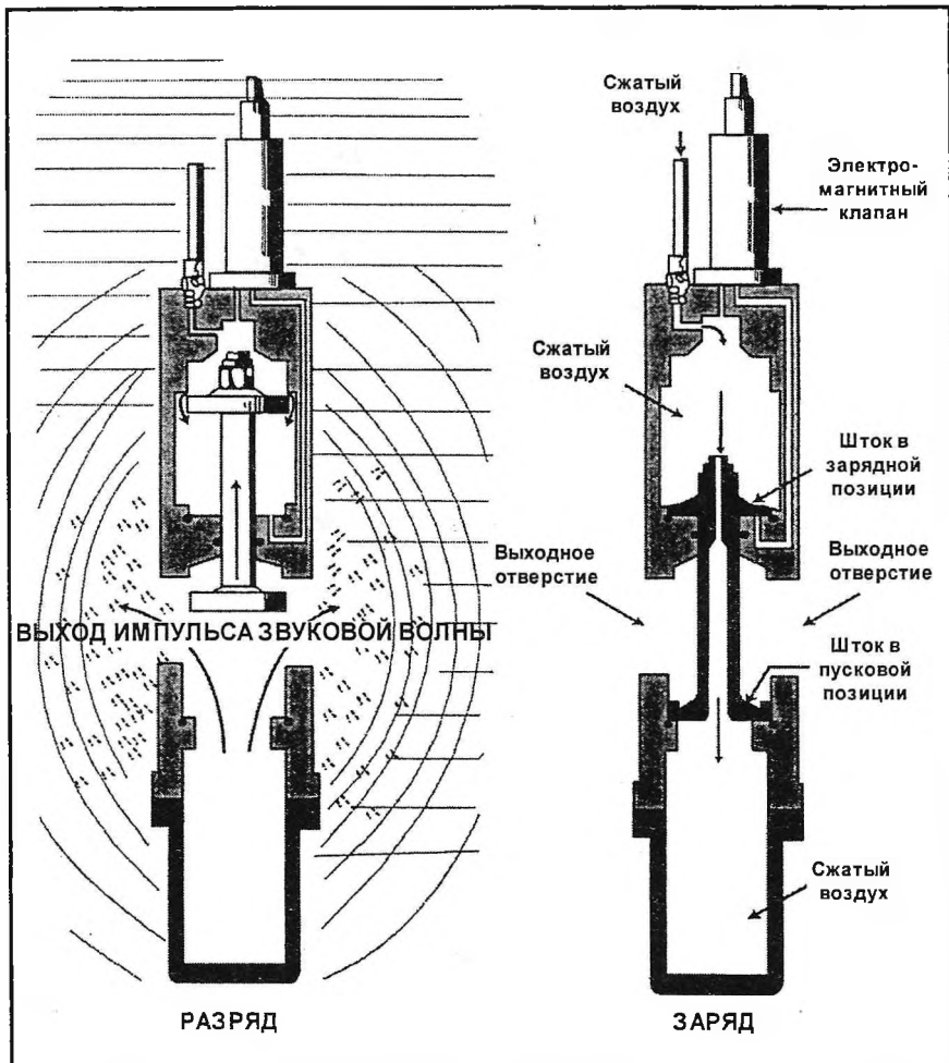
Рис. 2. Схема двухкамерного пневмоисточника упругих волн, применяемого в сейсморазведке
