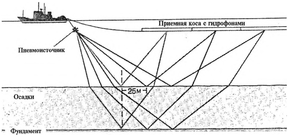
Рис. 1. Схема проведения сейсмопрофилирования на акватории
